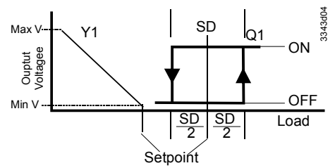
反向和正向动作顺序 (应用编号：50-59)
