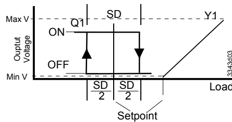
反向和正向动作顺序 (应用编号：40-49)
