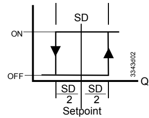
正向动作顺序 (应用编号：80-89)
