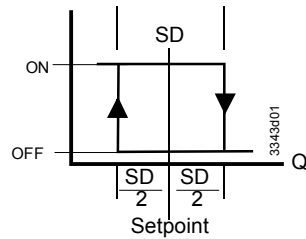
反向动作顺序 (应用编号：10-19)
